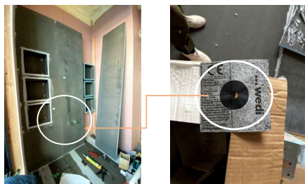
貫通パイプの防水カラーを設置
