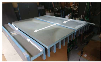
広い洗い場は3分割で搬入 排水路ユニット ／勾配床水下と水上
