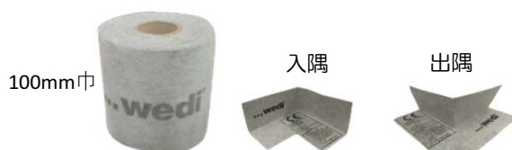
防水テープ(不織布製)
