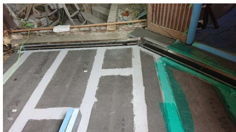
入口部のウェディボード貼りこみ ∧の字型の排水路は角度を合わせた 排水溝を工場で製作 レベルを合わせて現場で固定しました。
